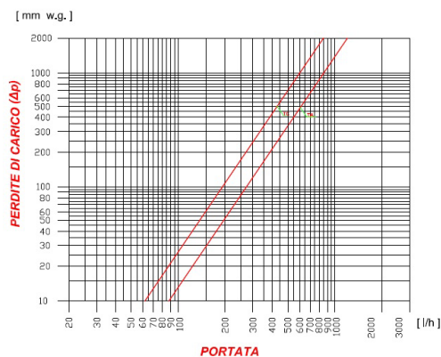
Valvola di zona Art.301 1" 82301AF05 DIAGRAMMA DELLE PERDITE DI CARICO
