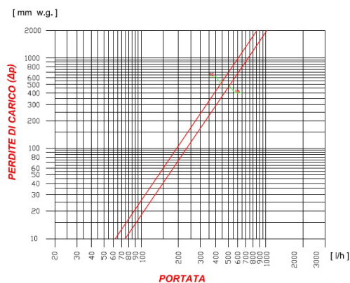
Valvola di zona Art.301 1/2" 82301AD05 DIAGRAMMA DELLE PERDITE DI CARICO
