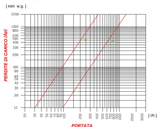
Valvola di zona Art.302 3/4" 82302AE05 DIAGRAMMA DELLE PERDITE DI CARICO
