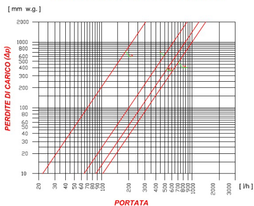
Valvola di zona Art.300 1" 82300AD05 DIAGRAMMA DELLE PERDITE DI CARICO
