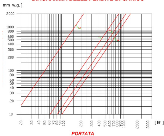
Valvola di zona Art.300 1/2" 82300AD05 DIAGRAMMA DELLE PERDITE DI CARICO
