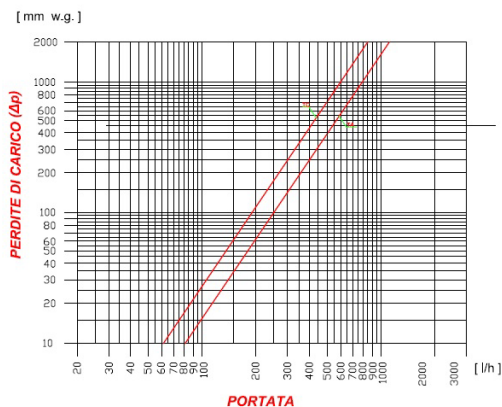
Valvola di zona Art.301 3/4" 82301AE05 DIAGRAMMA DELLE PERDITE DI CARICO
