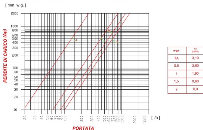
Valvola di zona Art.300 3/4" 82300AE05 DIAGRAMMA DELLE PERDITE DI CARICO
