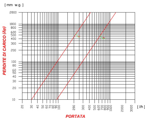
Valvola di zona Art.302 1/2" 82302AD05 DIAGRAMMA DELLE PERDITE DI CARICO
