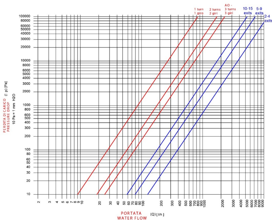
DIAGRAMMA DELLE PERDITE DI CARICO / PRESSURE DROP DIAGRAM
